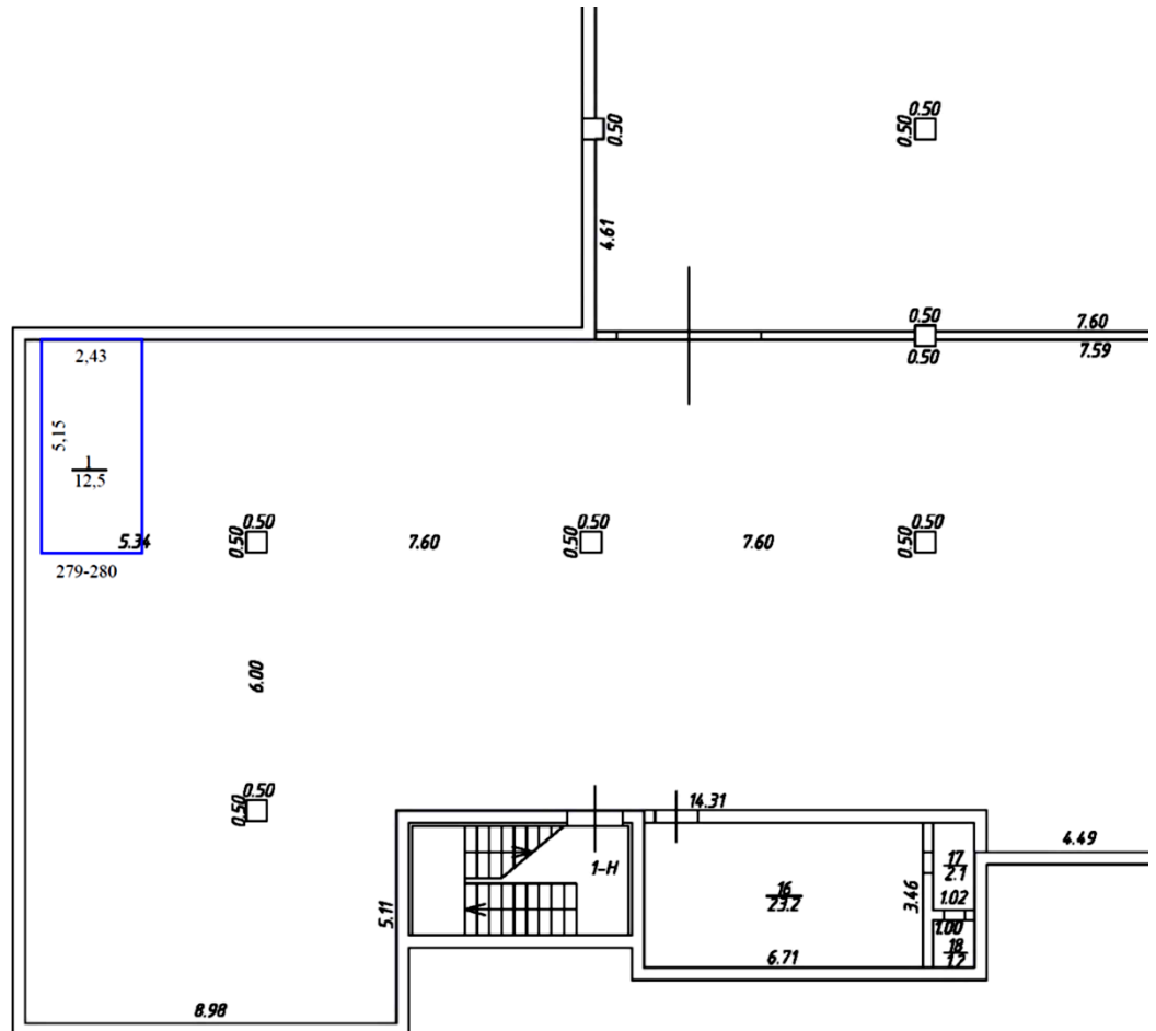
Фрагмент плана подвала
